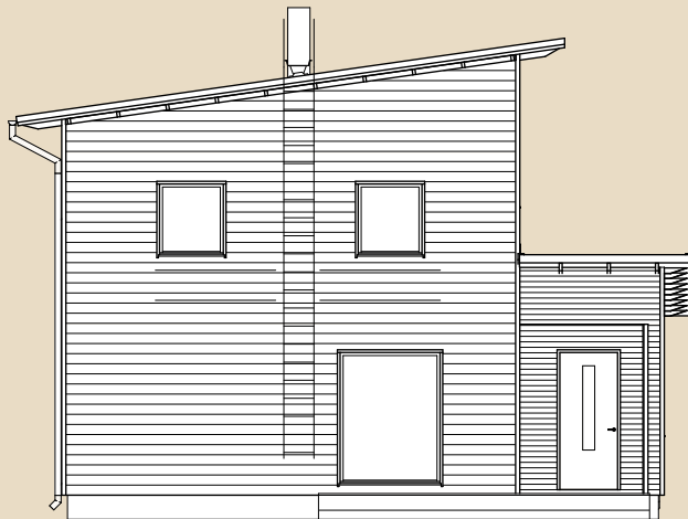
Eestvaade
