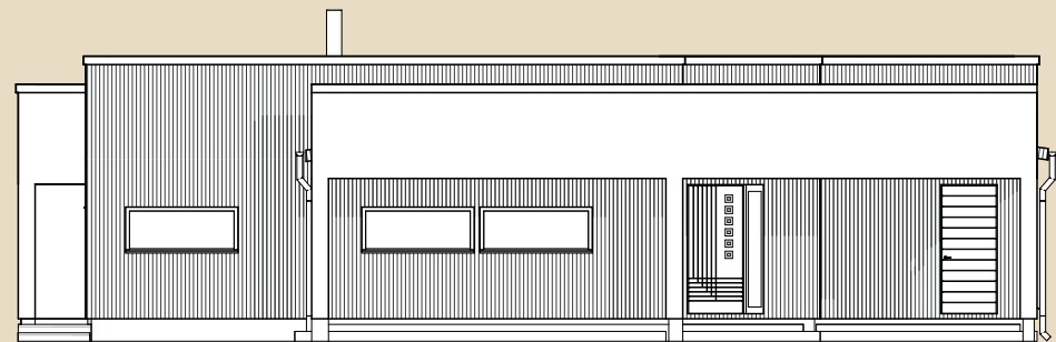
Vasak külg
