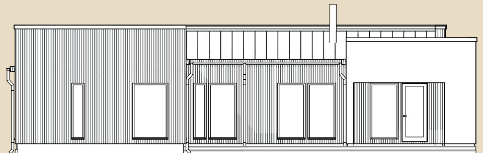
Parem külg
