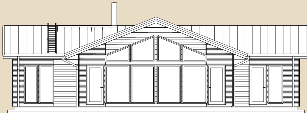
Tagantvaade
