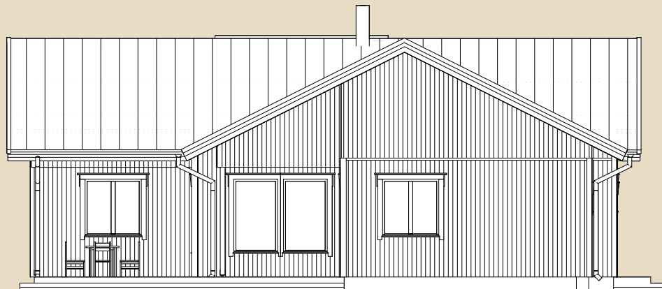
Tagantvaade
