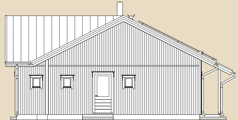
Vasak külg
