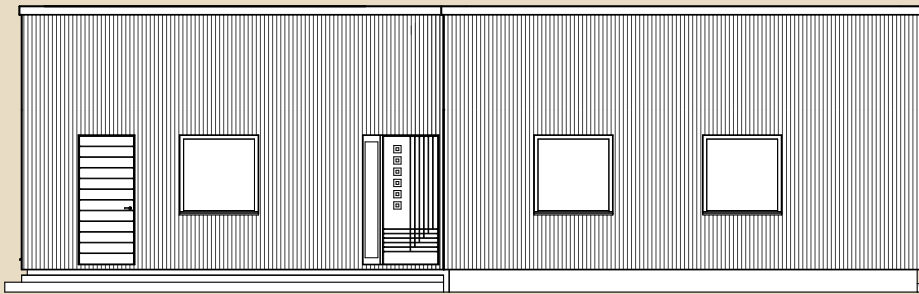
Eestvaade
