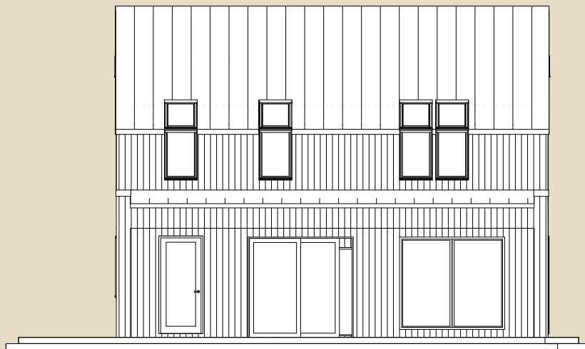
Tagantvaade
