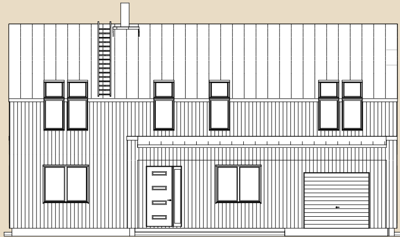
Eestvaade
