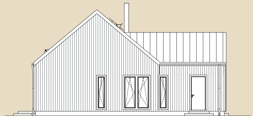
Parem külg
