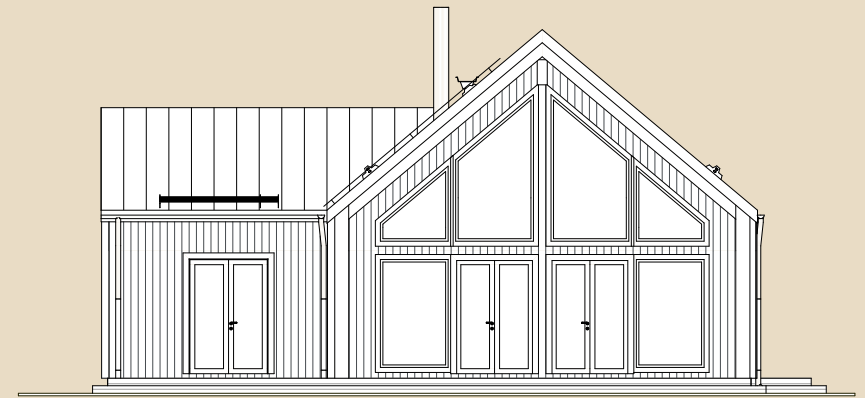
Vasak külg
