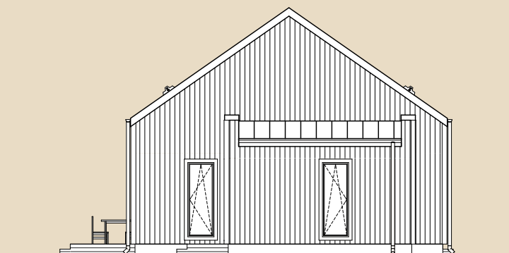
Parem külg
