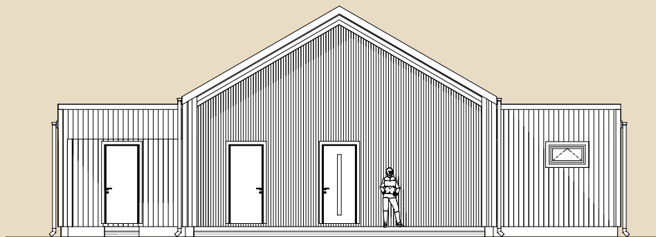
Eestvaade
