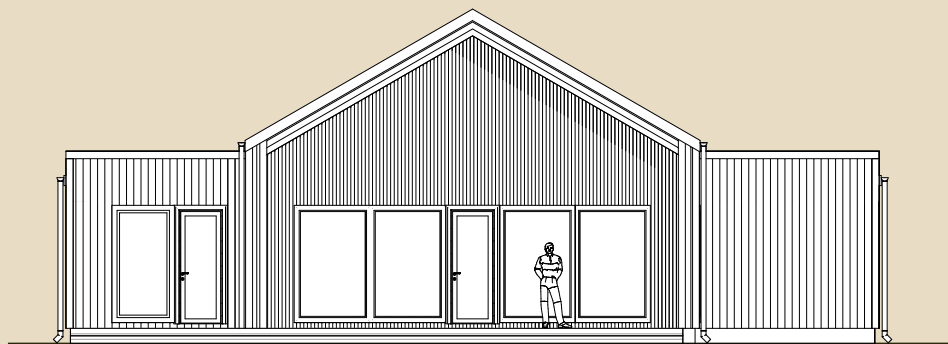
Tagantvaade
